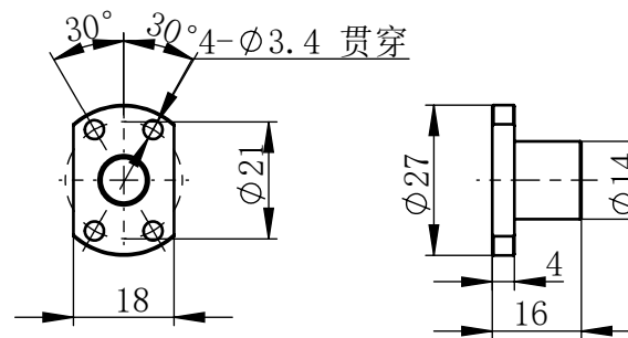
Nut
